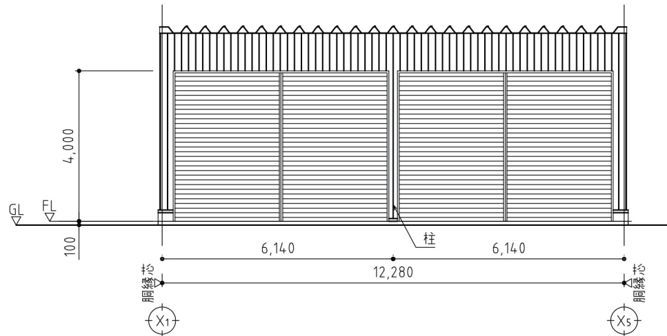
Y1 立面図
