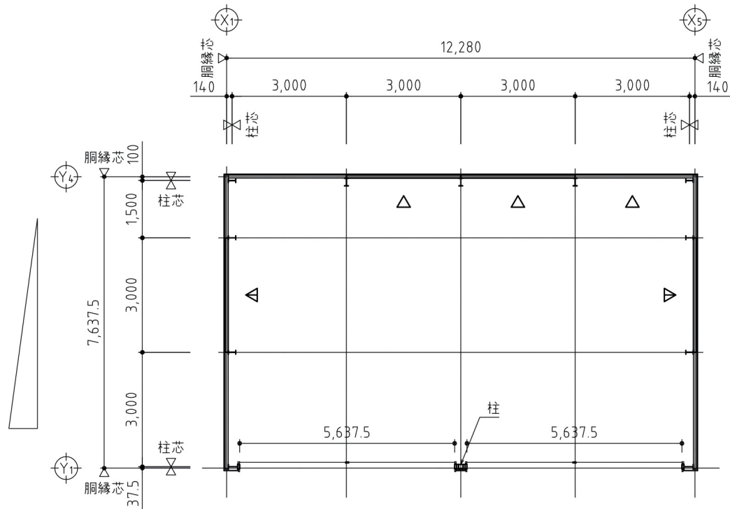
平面図
