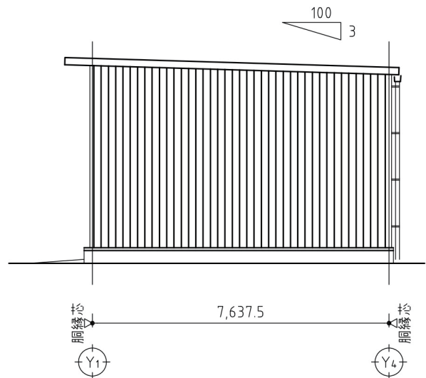
X5 立面図
