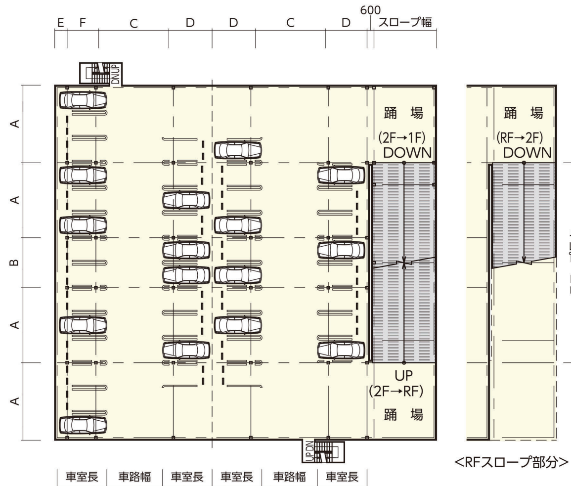
平面図 ※車室区画のWライン引きはオプション仕様です。
