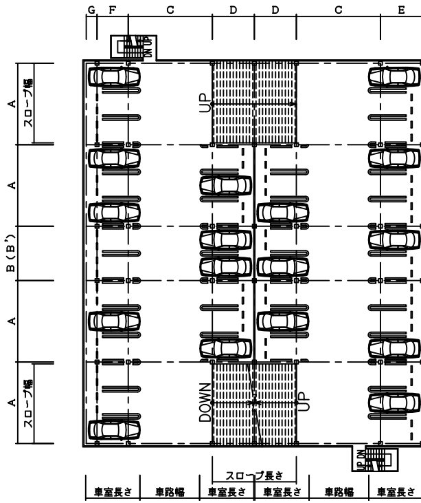
<2F平面図：NC-4N型/NC-4L型> ※車室区画のWライン引きはオプション仕様です。
